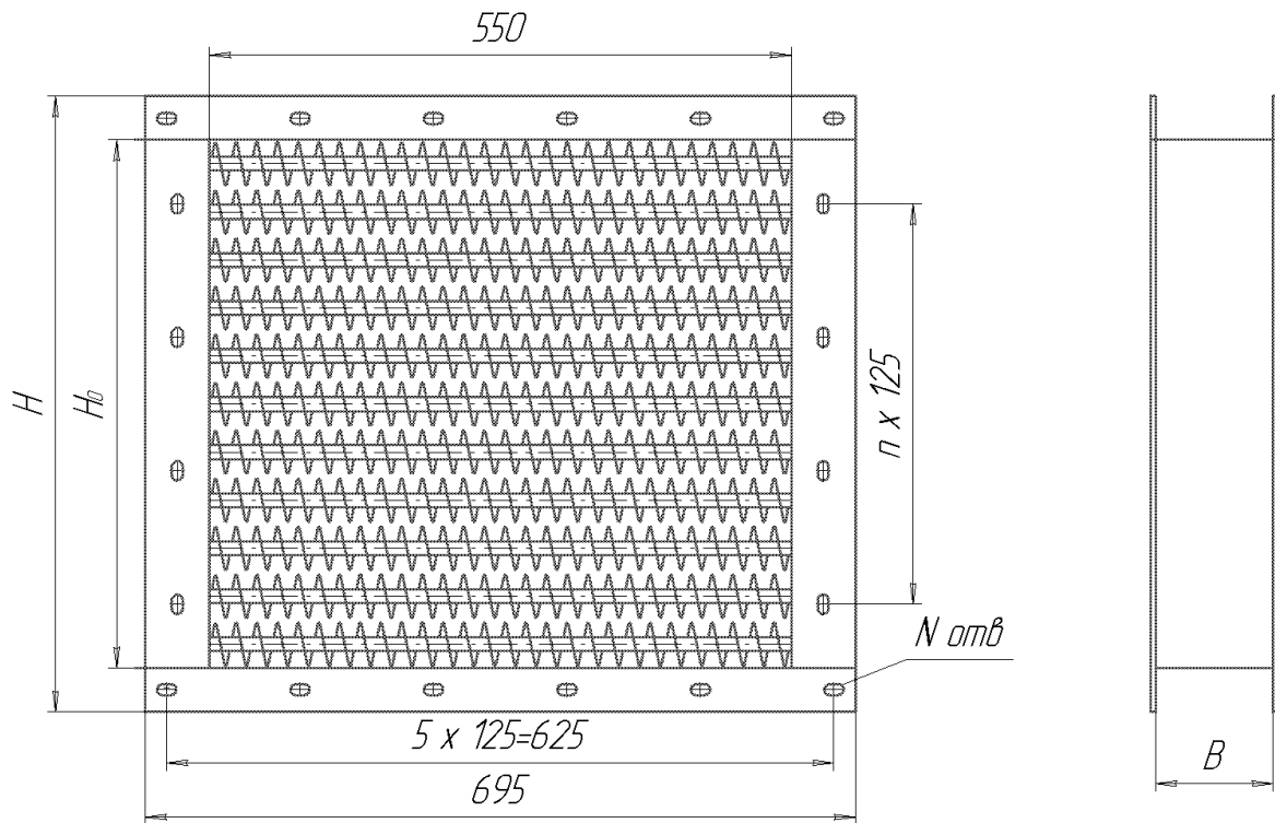
ГАБАРИТНЫЕ И ПРИСОЕДИНИТЕЛЬНЫЕ РАЗМЕРЫ, ММ
