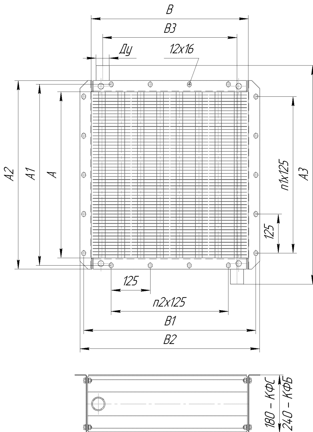
ГАБАРИТНЫЕ И ПРИСОЕДИНИТЕЛЬНЫЕ РАЗМЕРЫ КАЛОРИФЕРОВ КФС; КФБ.
