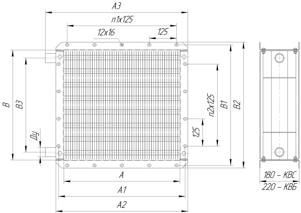
ГАБАРИТНЫЕ И ПРИСОЕДИНИТЕЛЬНЫЕ РАЗМЕРЫ КАЛОРИФЕРОВ КВС и КВБ.
